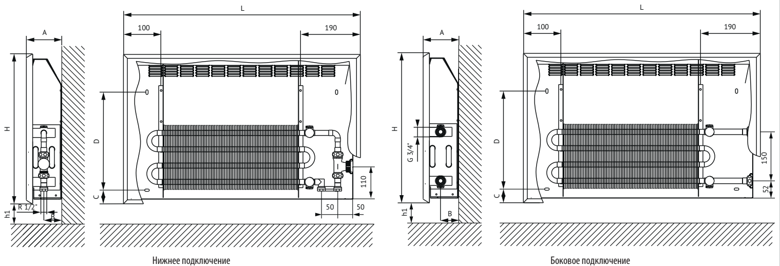
Нижнее подключение
